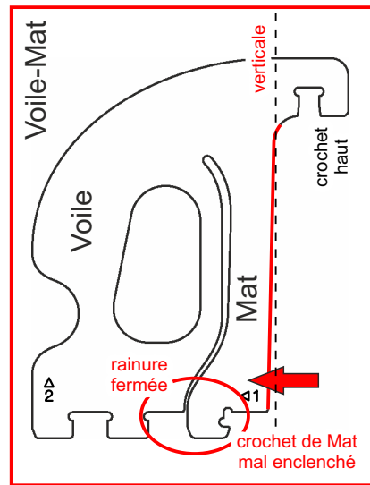
Voile-Mat mal montée La cale n'entre pas dans la rainure
