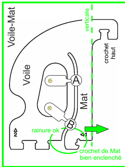
Voile-Mat bien montée La cale rentre dans la rainure
